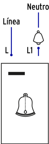
Diagrama de conexión
