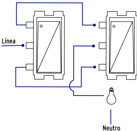
Diagrama de conexión
