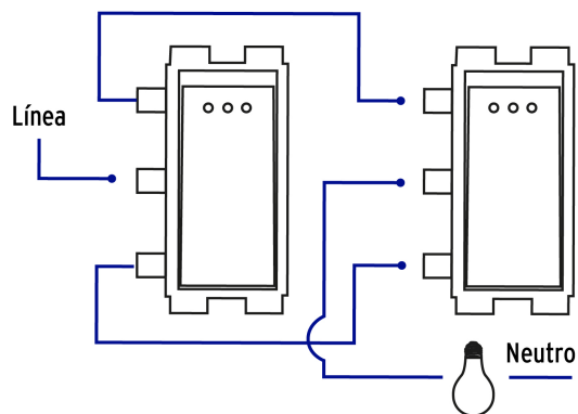
Diagrama de conexión
