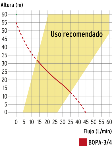
Curva de rendimiento periféricas autocebantes
